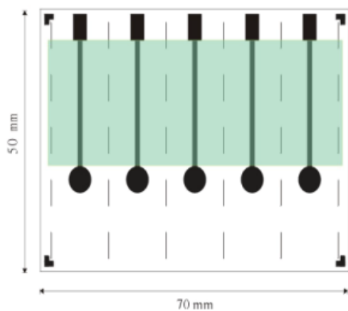
圖 2 網版印刷電極組成示意圖 (a)網版印刷單電極全貌； (b)網版印刷電極剖面圖
