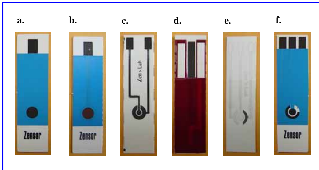
圖 1 不同類型網版印刷電極 a.網版印刷單電極； b.奈米銅網版印刷電極； c.環盤印刷電極； d.超微網版印刷電極； e.銀膠三電極； f.三電極電化學試片。
