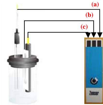
圖 3 試片示意圖 (a)參考電極； (b)工作電極； (c)輔助電極
