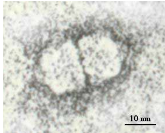
圖、雙生病毒電子顯微鏡圖
