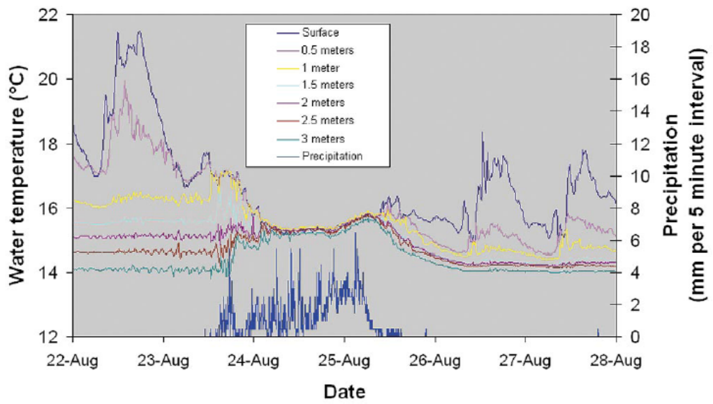
圖 1 颱風帶來的大量降雨對不同深度的水溫所造成的變化
