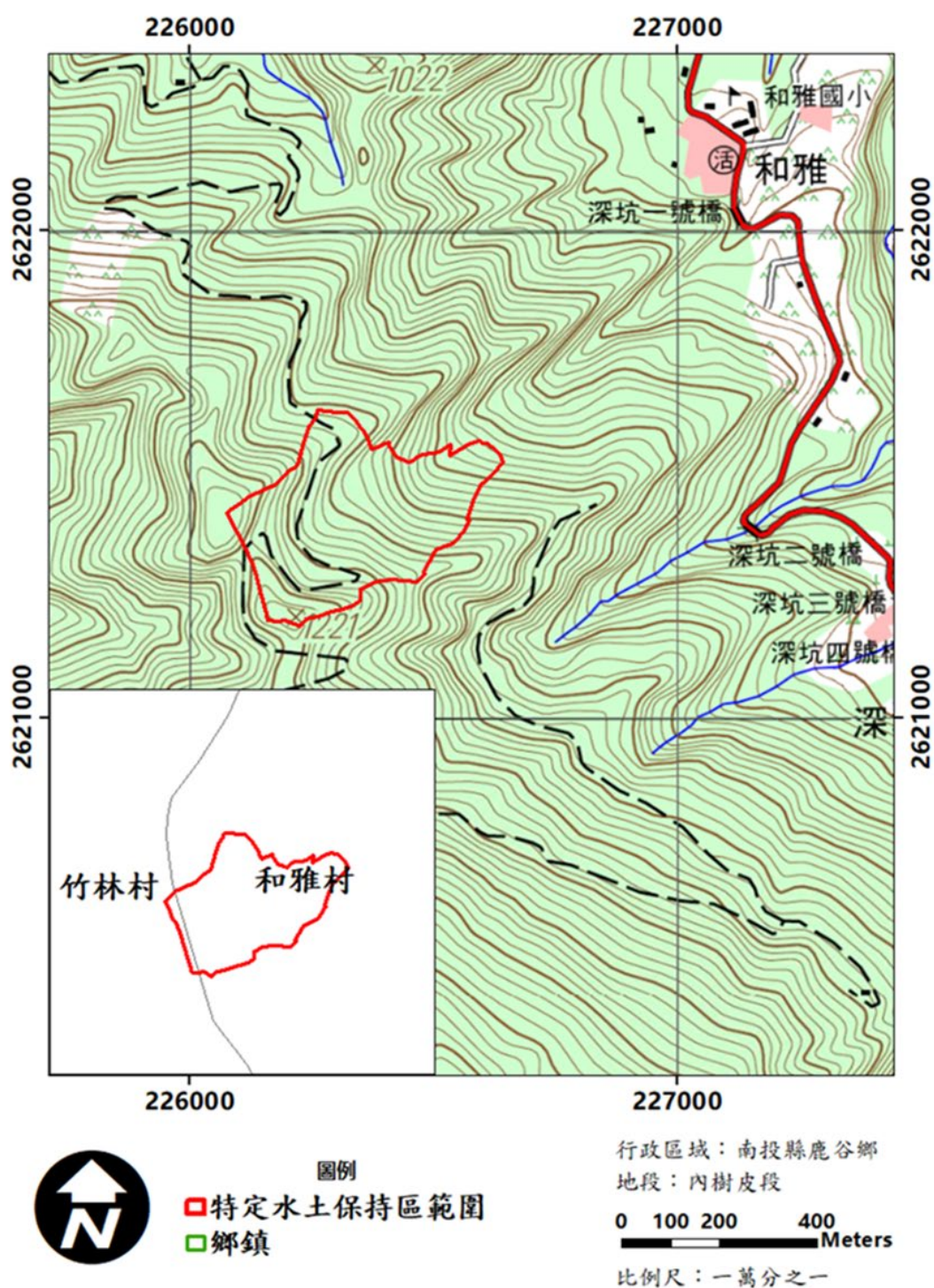
南投縣鹿谷鄉LL004和雅內高大規模崩塌特定水土保持區位置圖
